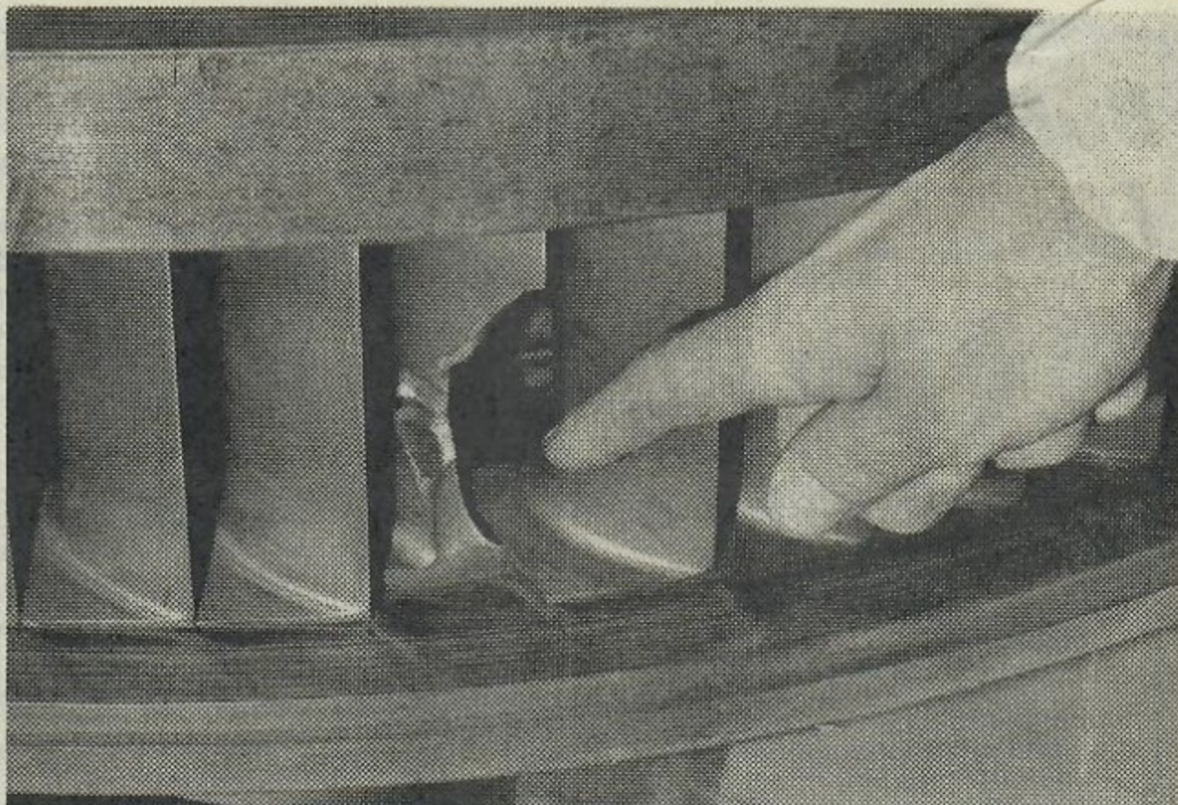
Mycket kan hända i ett kärnkraftverk. Allt behöver dock inte innebära katastrof. Här ett brott på ett skovelblad i turbinen på »Oskar I».
